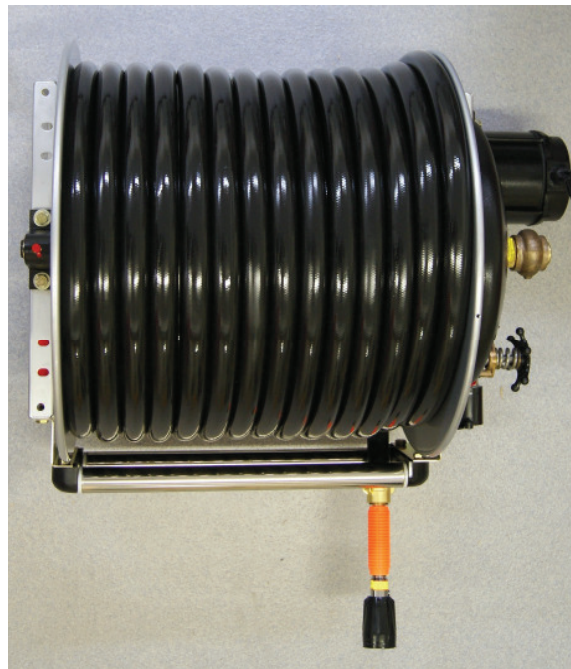
Abbildung mit 60m 25/34mm Schlauch
